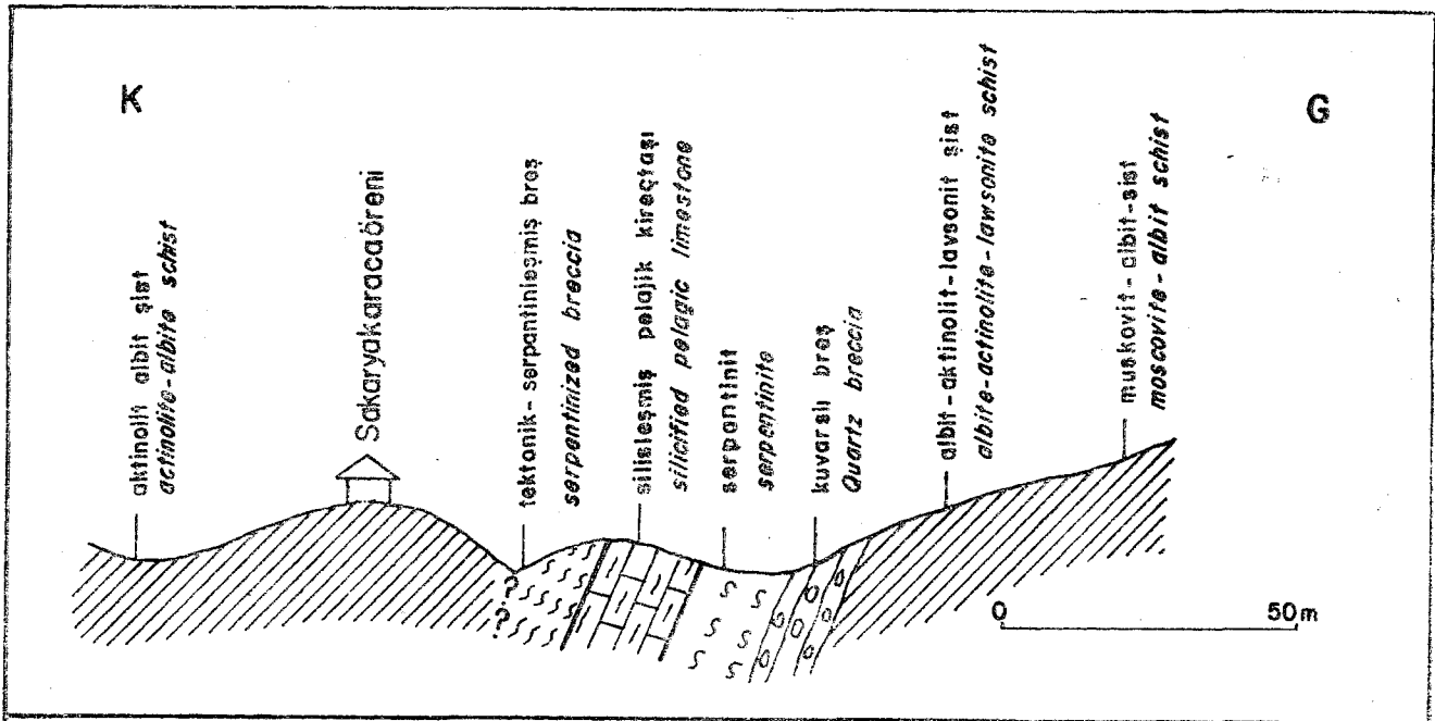
Şekil 4: Sakarya kuzeyi, Sakaryakaracaöreni'nden geçen enine kesit.
