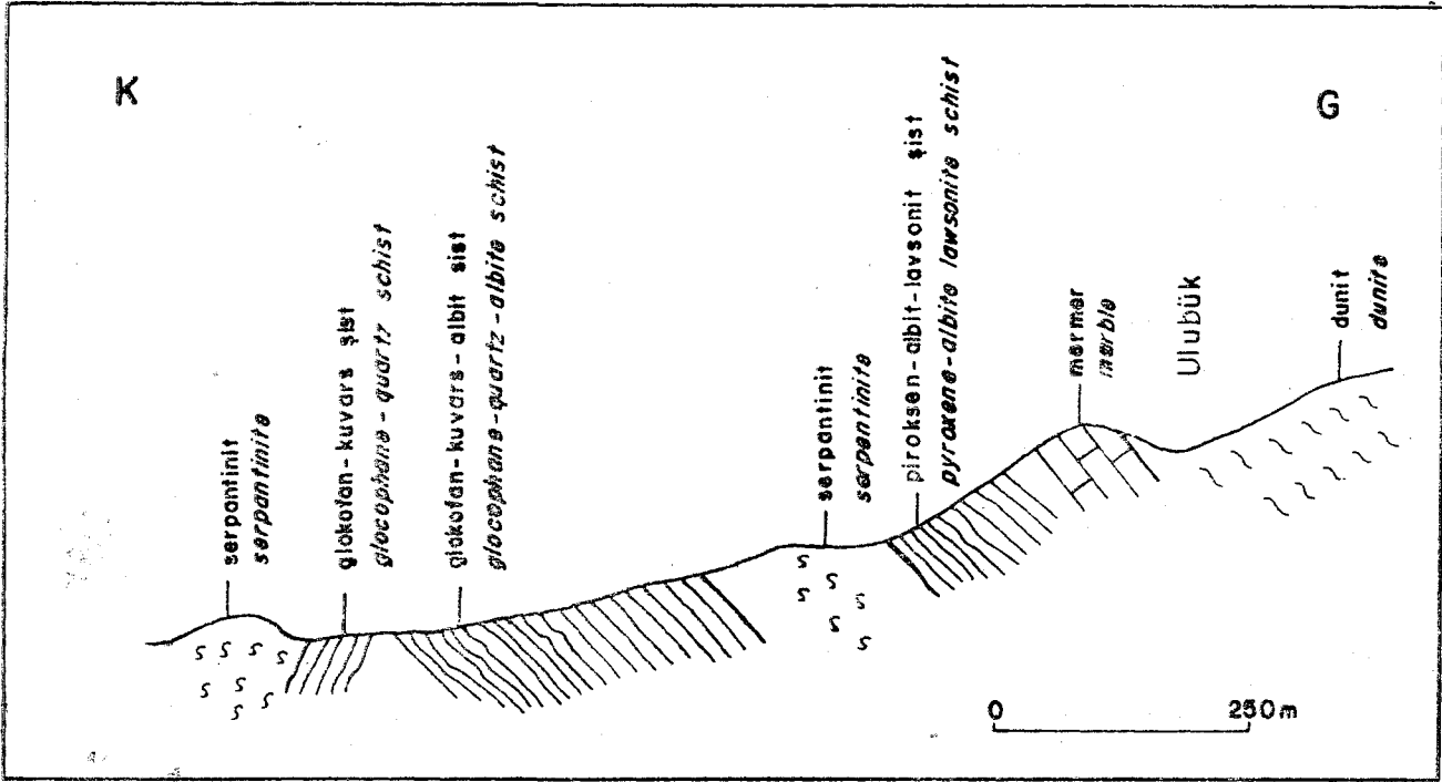
Sekli 5: İnceleme alan doğusunda Ulubük'ten geçen enine kesit.
