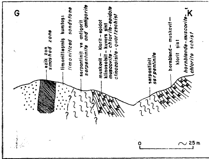
Şekil 8: Bilecik güneyi, Demirköy'ün yaklaşık 1 km kuzeyinde Karasu kenarından geçen enine kesit; serpantini* ve antigoritlerin, yeşilistlerle dokanak ilişkileri.
