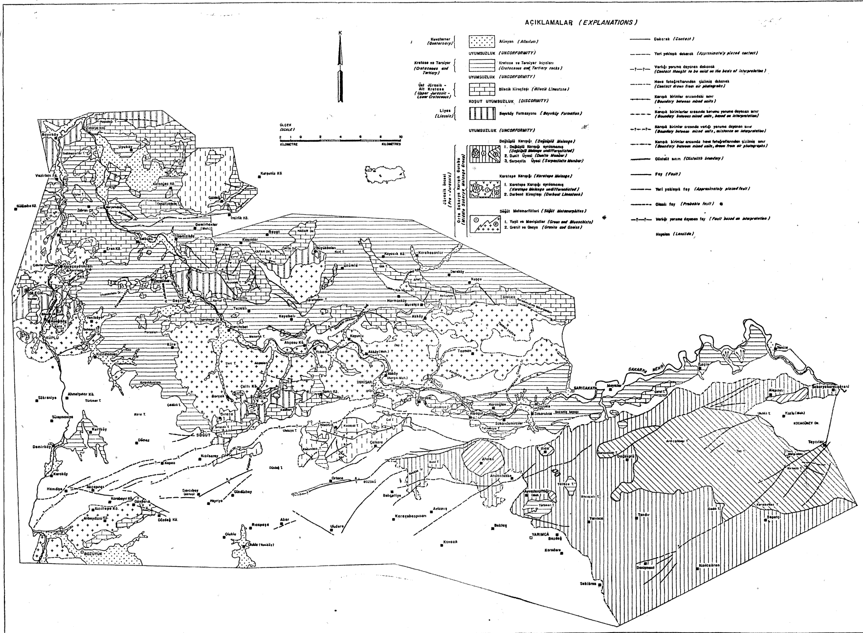
Şekil 2: Bilecik-Gökçekaya barajı arasındaki alanın sadeleştirilmiş jeoloji haritası. Figure 2: The simplified geological map of the area between Bilecik and Gökçekaya Dam.
